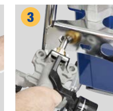
3 A hatlapfejű rögzítőelemmel lazítsa ki a szivattyút, és vegye ki az egységet
