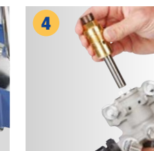
4 Cserélje ki a szivattyút, és tegye vissza az egységet
